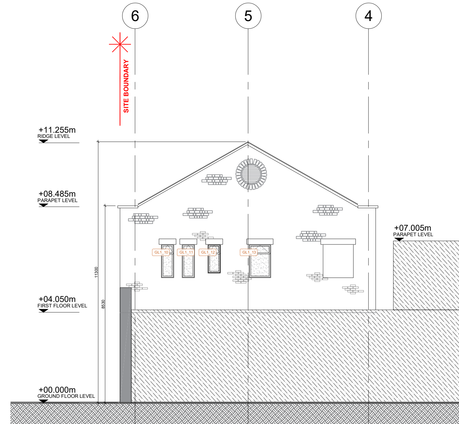
5 30.00 WEST ELEVATION SCALE: 1:100
